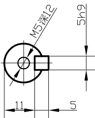
轴端剖面 A-A Shaft end section
