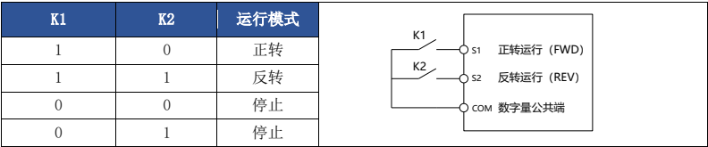
图 6-9 两线式模式 2
