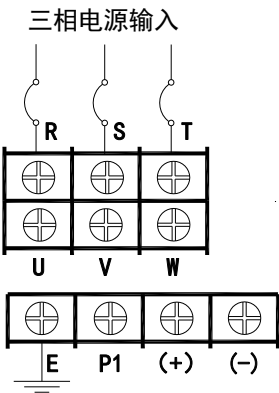
j) 500kW-630kW 变频器主回路端子排配线图
