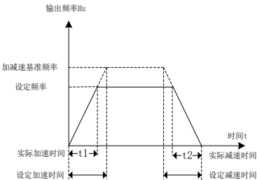
图 6-3 加减速时间示意图
