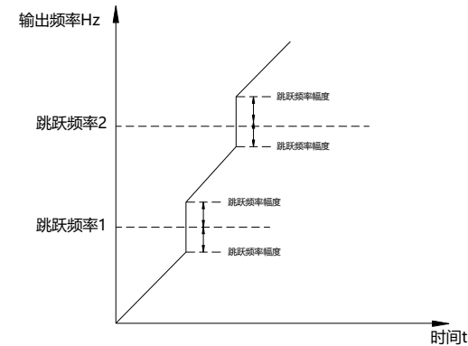
图 6-18 加减速过程中跳跃频率有效示意图
