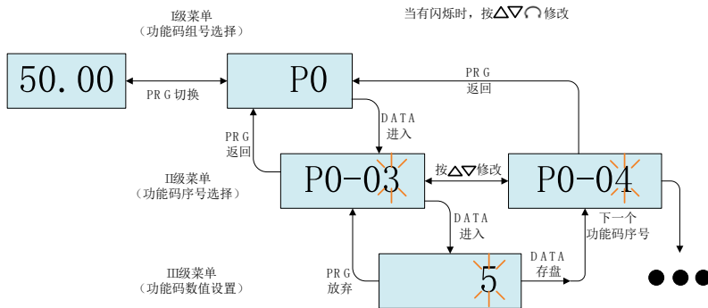
图 4-2 三级菜单操作流程圖
