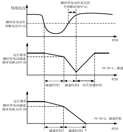
图 6-24 瞬时停电动作示意图
