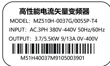
图 2-2 铭牌
