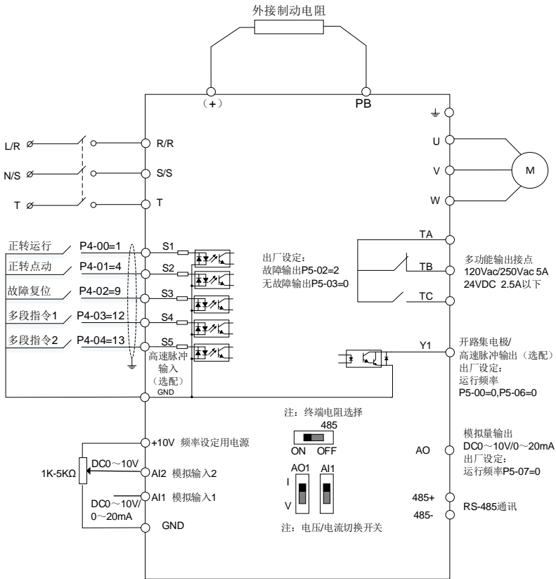
图 3-4 标准接线图
