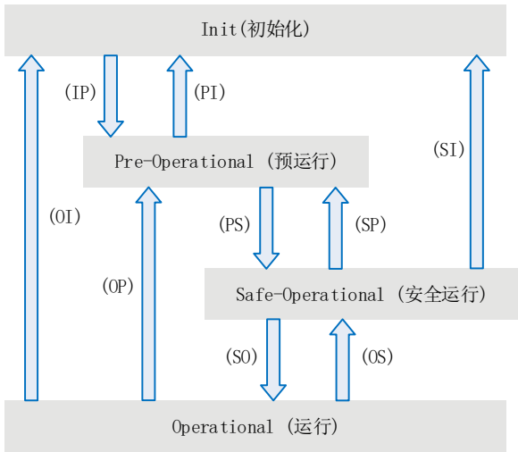
图 6-4 EtherCAT 状态机
