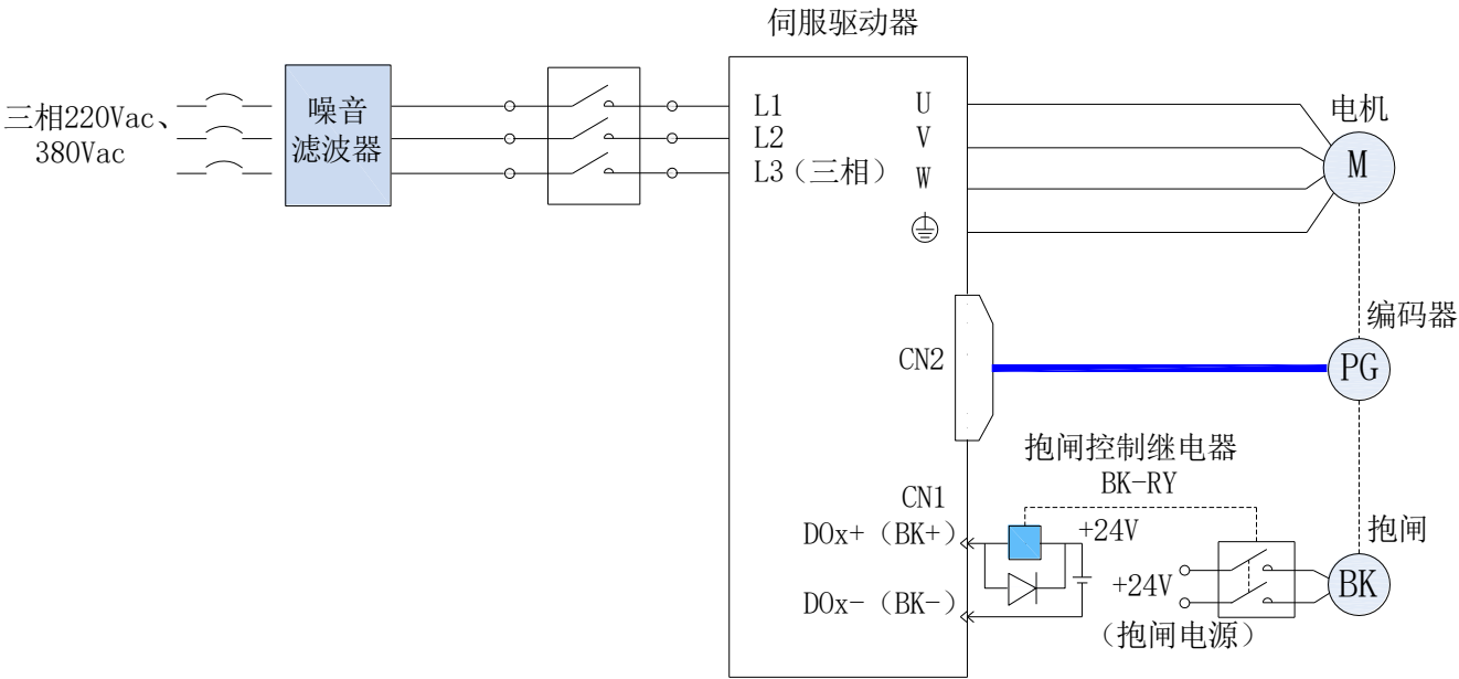
图 7-4 抱闸配线图
