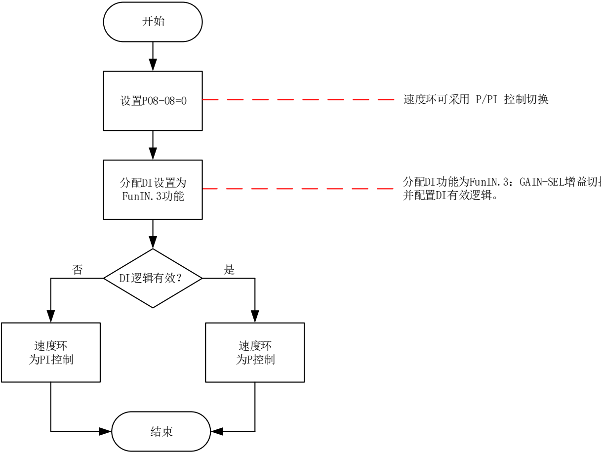
图 9-7 P08-08=0 增益切换流程图
